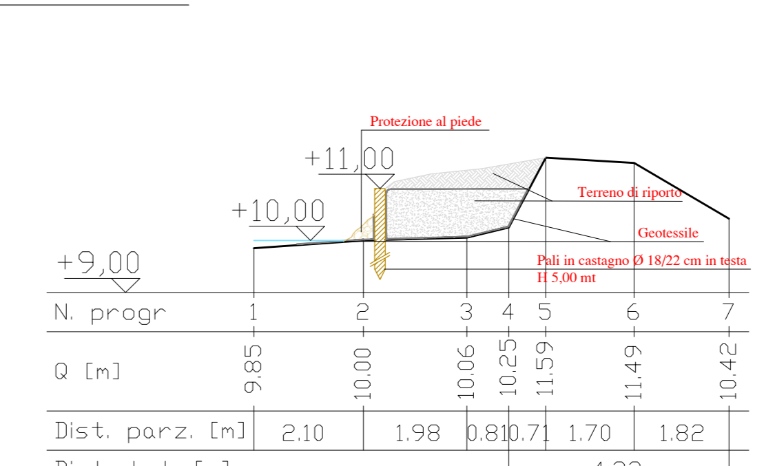
SEZIONE 18 - STATO DI PROGETTO - SCALA 1:100
