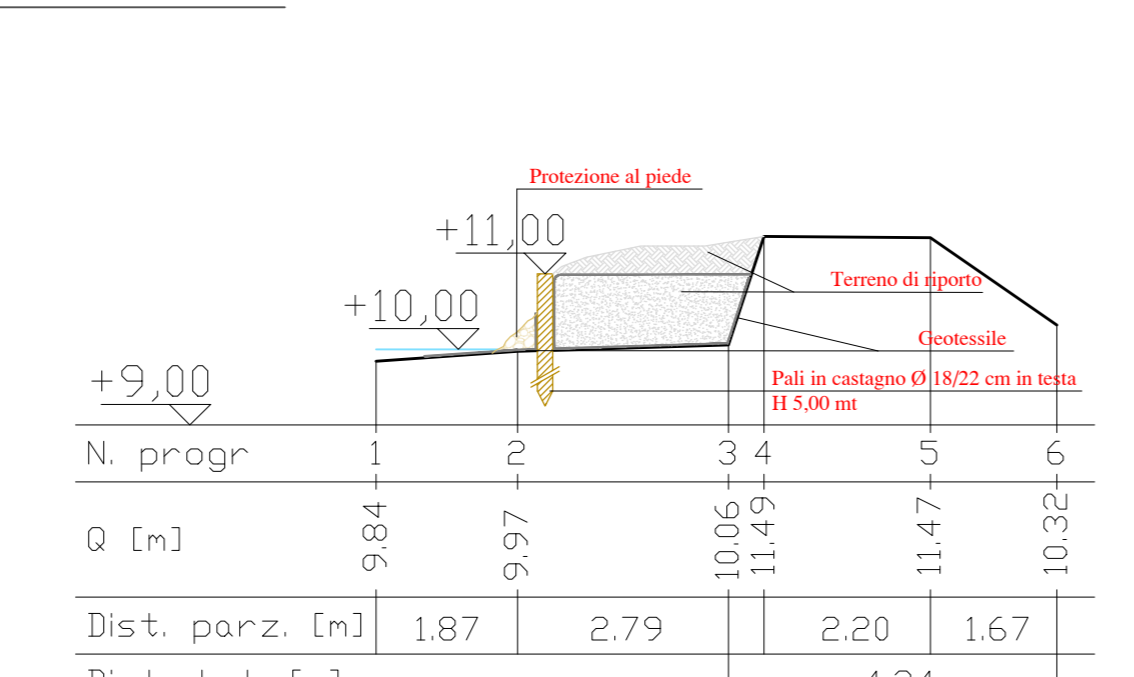
SEZIONE 17 - STATO DI PROGETTO - SCALA 1:100
