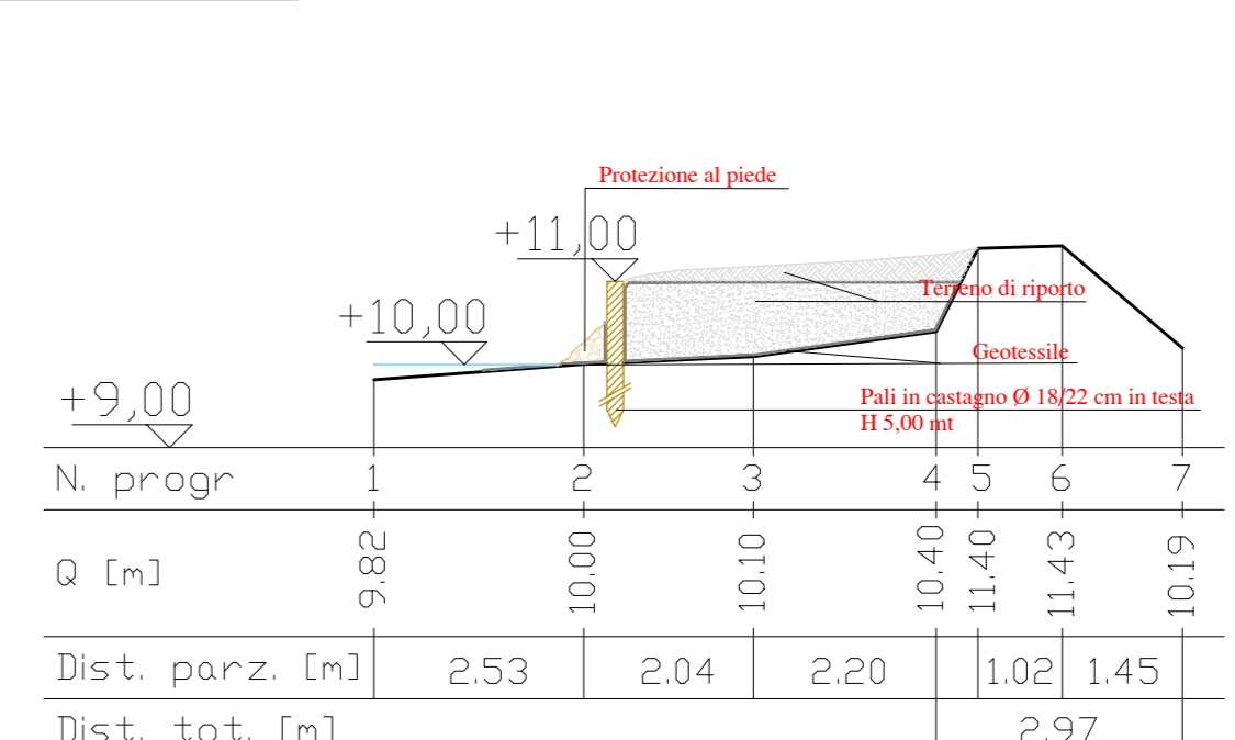
SEZIONE 16 - STATO DI PROGETTO - SCALA 1:100
