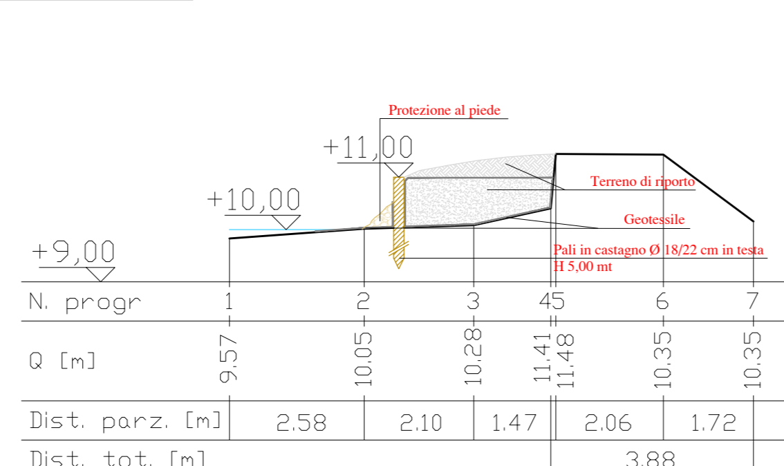
SEZIONE 15 - STATO DI PROGETTO - SCALA 1:100
