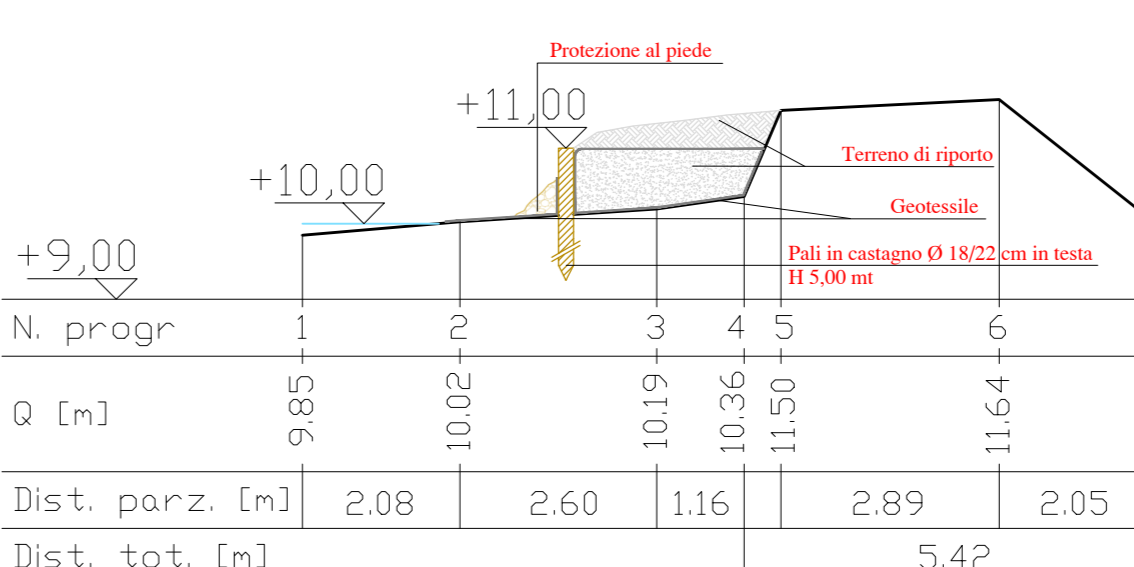
SEZIONE 14 - STATO DI PROGETTO - SCALA 1:100
