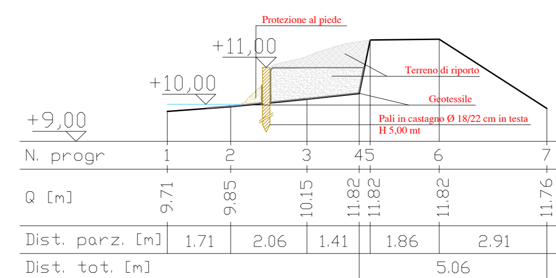
SEZIONE 10 - STATO DI PROGETTO - SCALA 1:100
