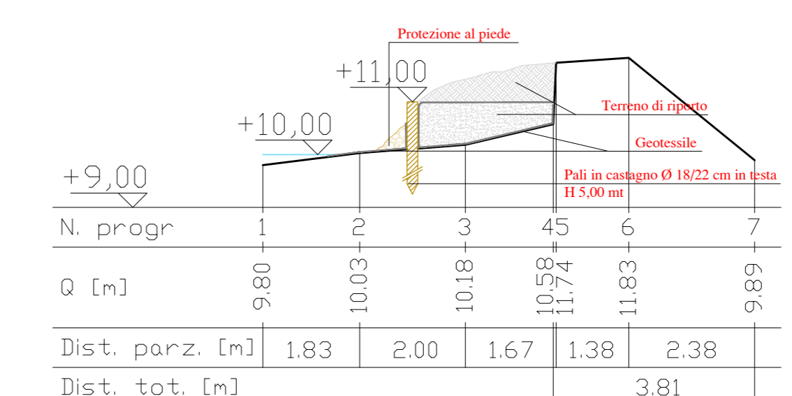
SEZIONE 11 - STATO DI PROGETTO - SCALA 1:100
