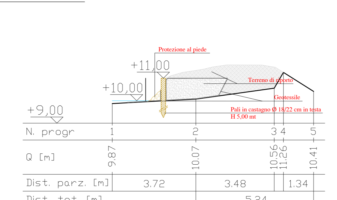
SEZIONE 19 - STATO DI PROGETTO - SCALA 1:100
