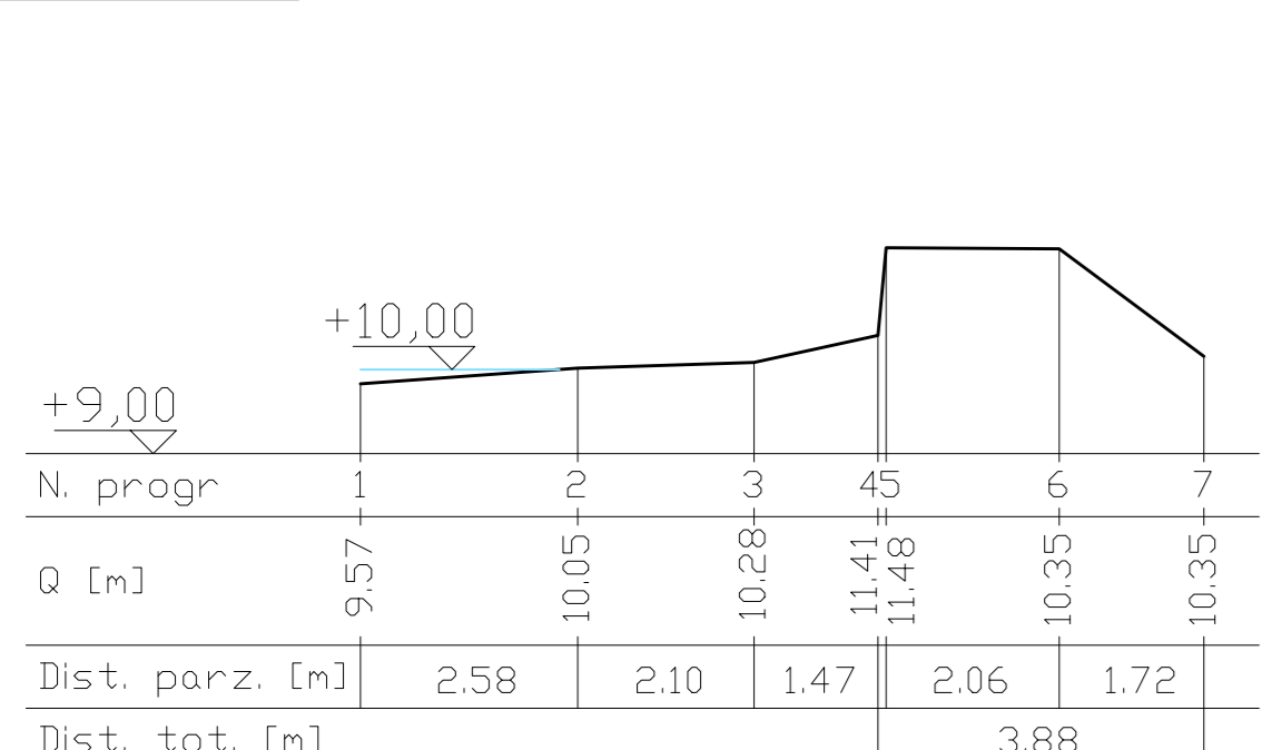
SEZIONE 15 - STATO DI FATTO - SCALA 1:100
