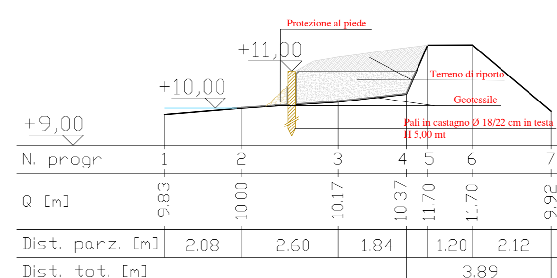
SEZIONE 13 - STATO DI PROGETTO - SCALA 1:100
