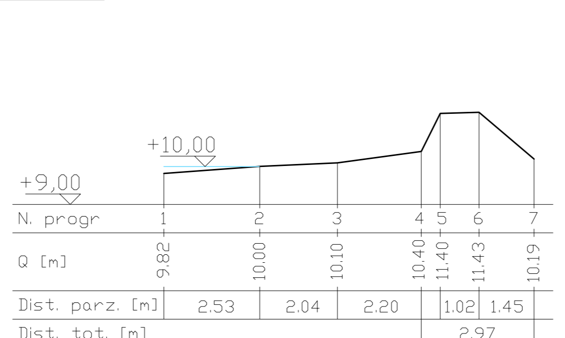
SEZIONE 16 - STATO DI FATTO - SCALA 1:100
