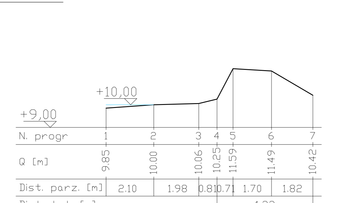
SEZIONE 18 - STATO DI FATTO - SCALA 1:100
