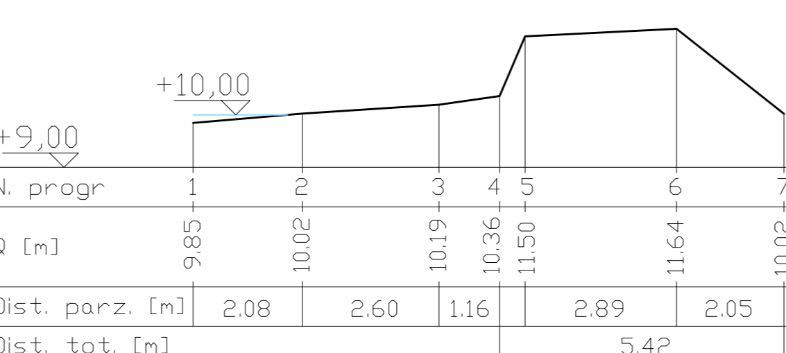
SEZIONE 16 - STATO DI FATTO - SCALA 1:100
