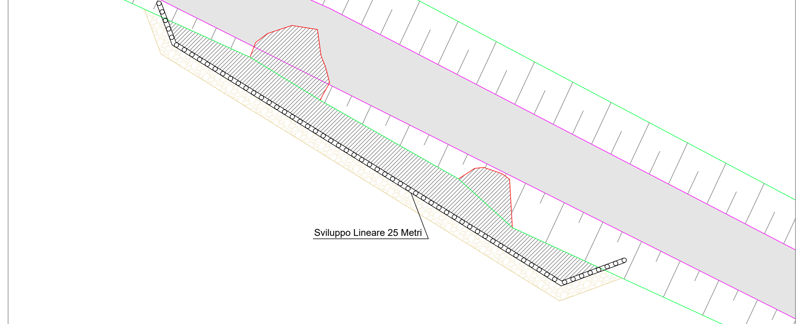
PARTICOLARE SEZIONE 21 - SCALA 1:100
