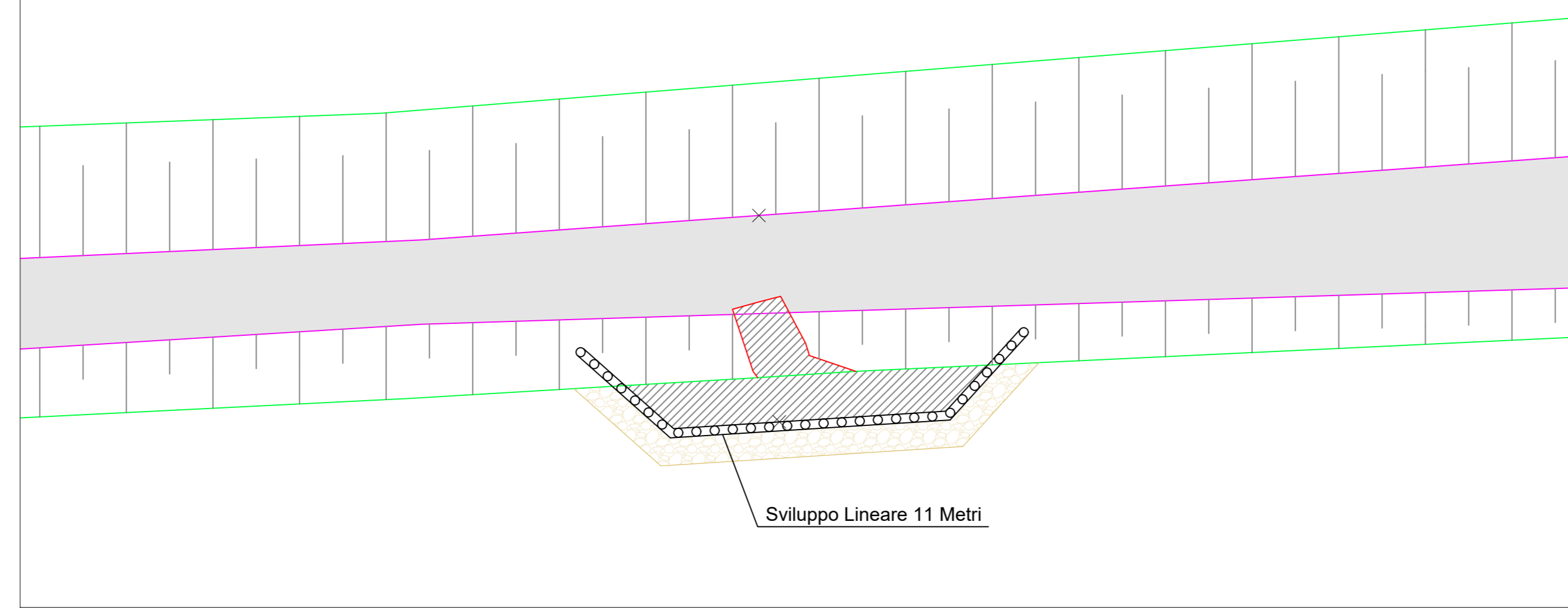
PARTICOLARE SEZIONI 15-16-17-18-19-20 - SCALA 1:200
