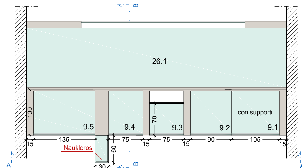
SEZIONE B
