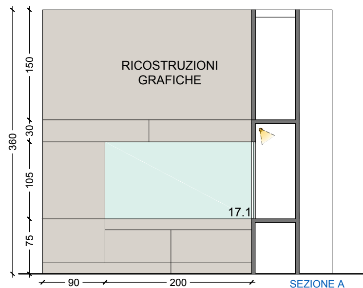
SEZIONE A
