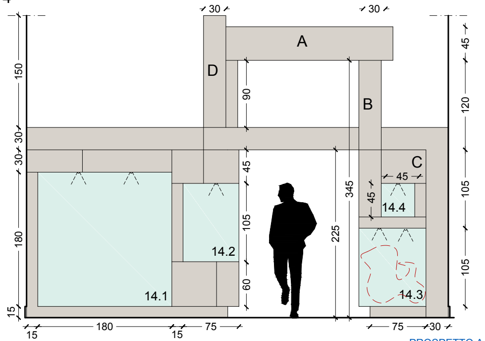
PROSPETTO A
