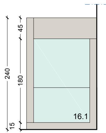
SEZIONE A
