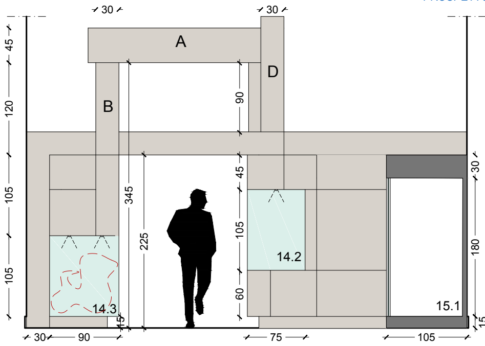
SEZIONE D
