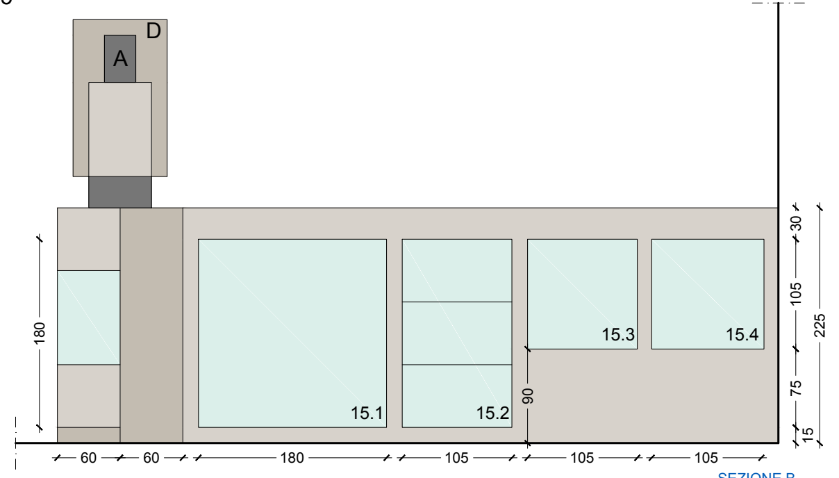
SEZIONE B
