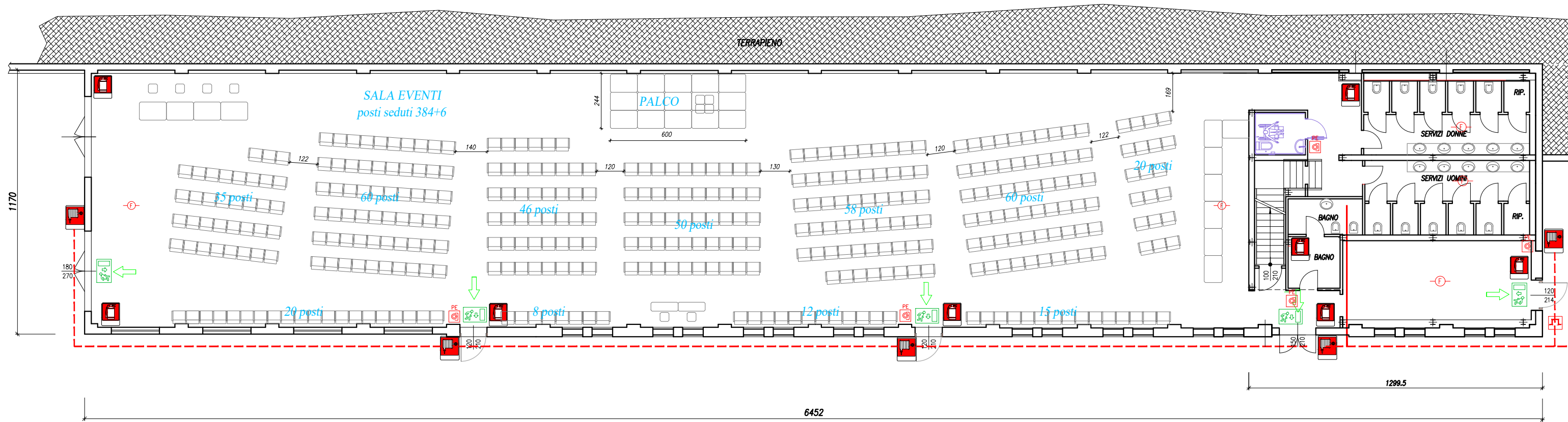
PIANTA PIANO TERRA (CROGIOLO) (SCALA 1:100)
