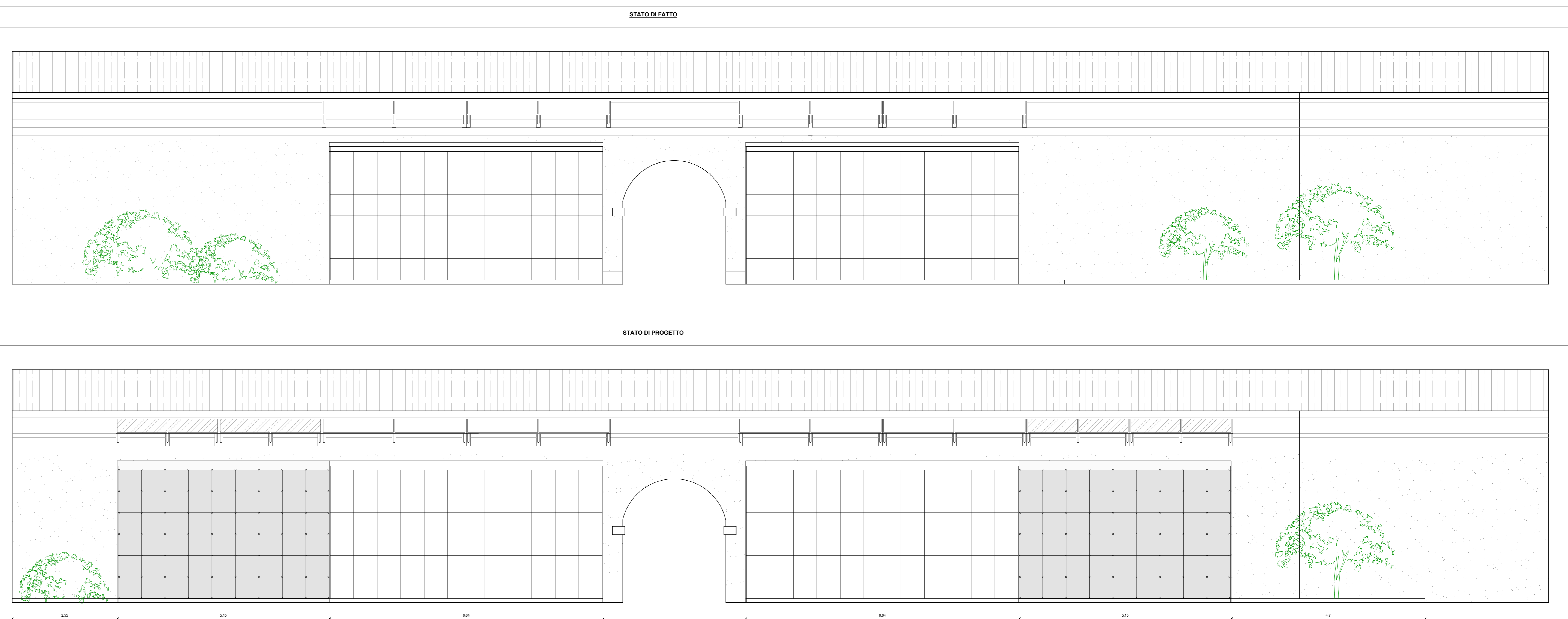
PROSPETTO FRONTALE - scala 1:50
