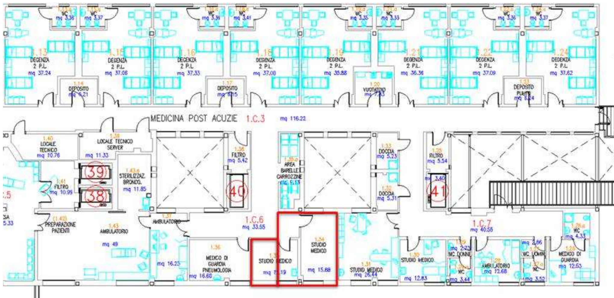
Ipotesi di layout dei locali (st. 1.34-1.35) per installazione diagnostica radiologica
