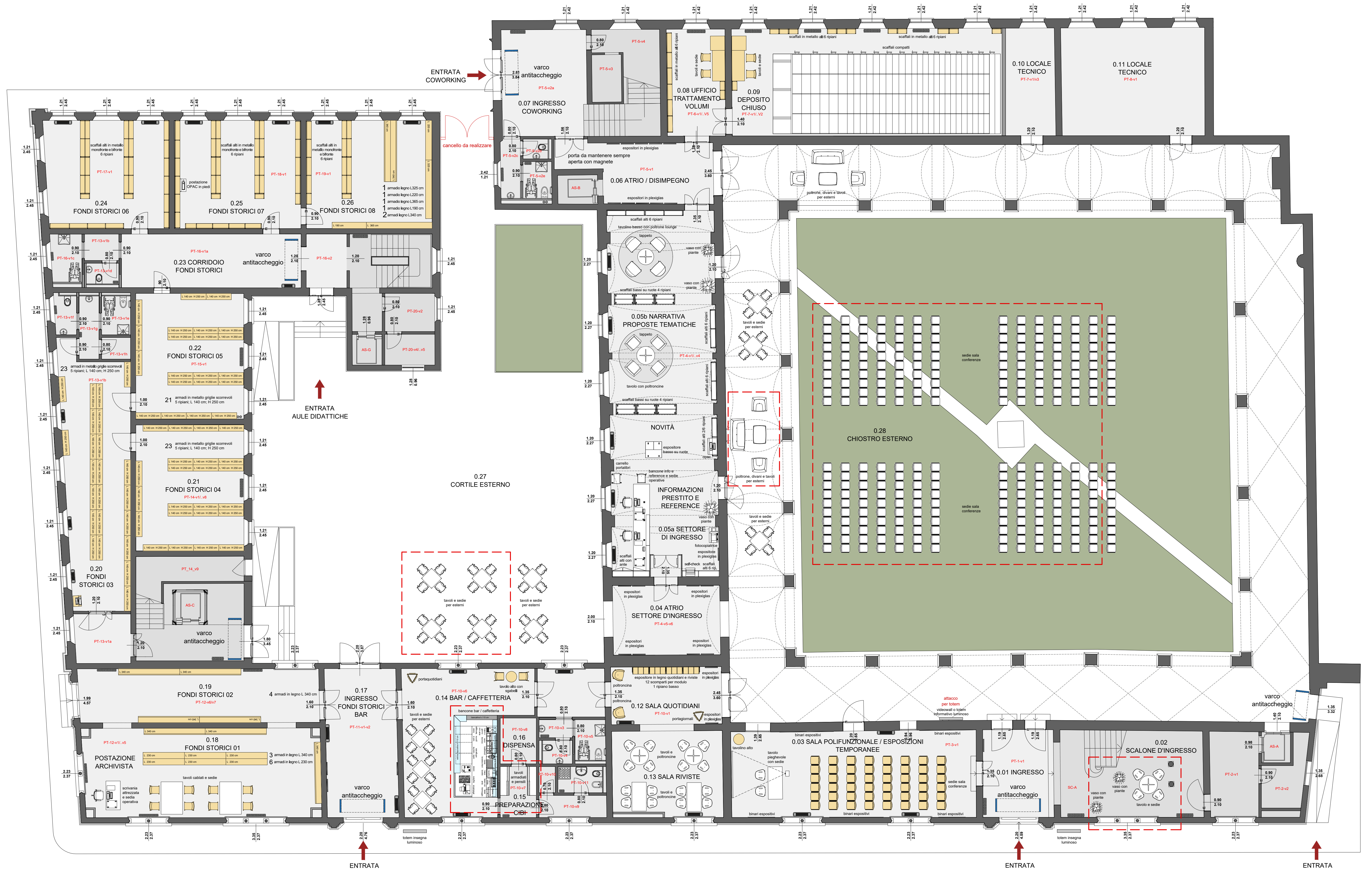
PIANTA ARREDATA PIANO TERRA scala 1:100
