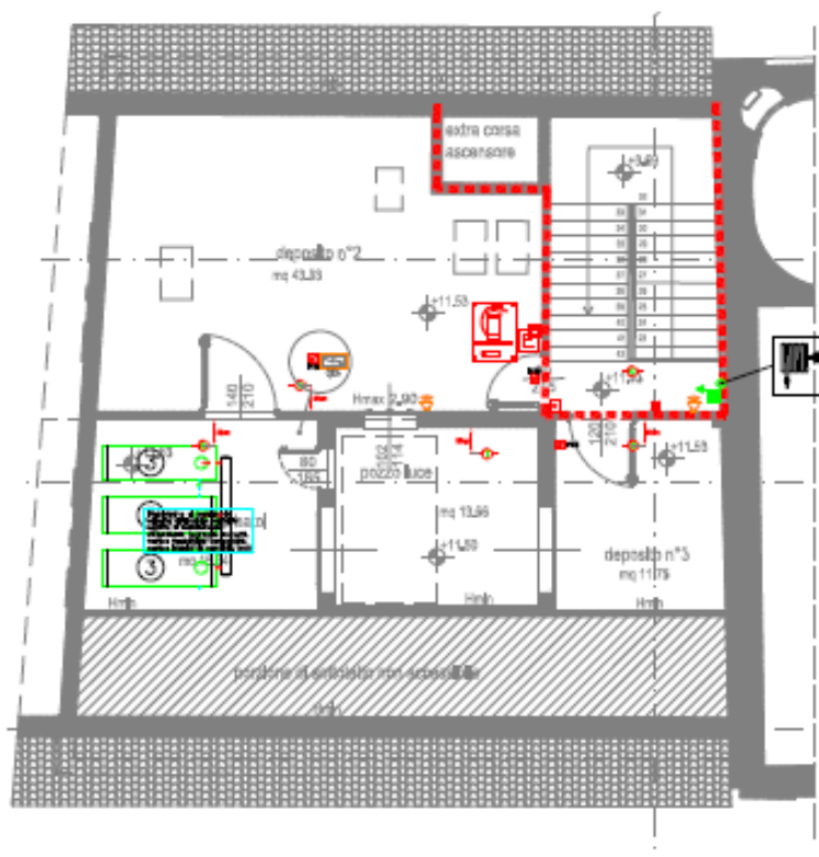
Planta sottotetto Scala 1:100
