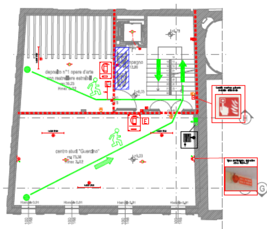
Planta piano secondo ammezzato Scala 1:100
