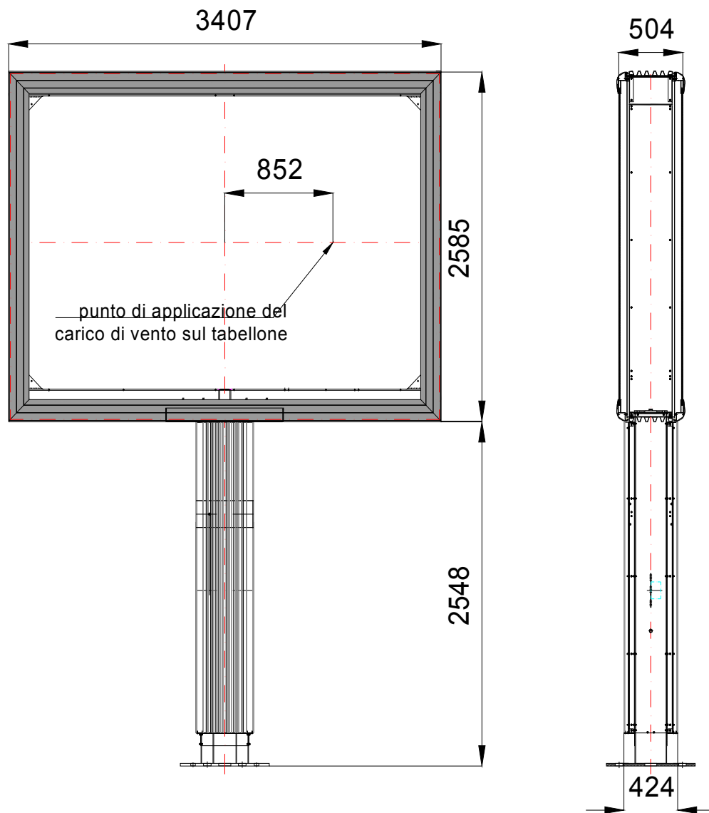
Illustrazione 1: dimensioni del pannello e punto di applicazione di calcolo per il carico di vento
